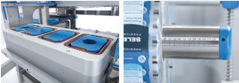
Snelle wisseling van folie en formaatdeel zonder gebruik van gereedschap
