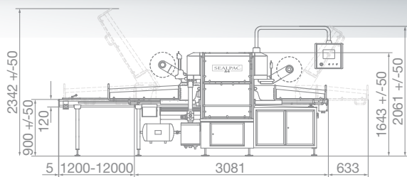
Ca. 30 schalen/minuut
