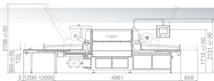
Ca. 200 schalen/minuut
