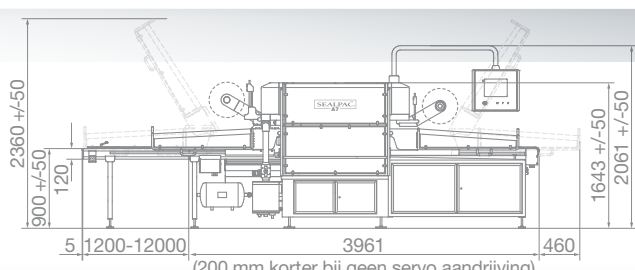
Ca. 100 schalen/minuut
